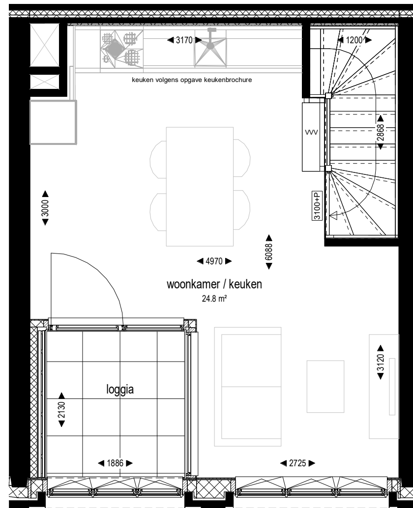
VERDIEPING 1
